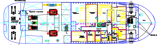
План главной палубы и палубы пассажира
