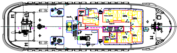
План главной палубы и палубы пассажира
